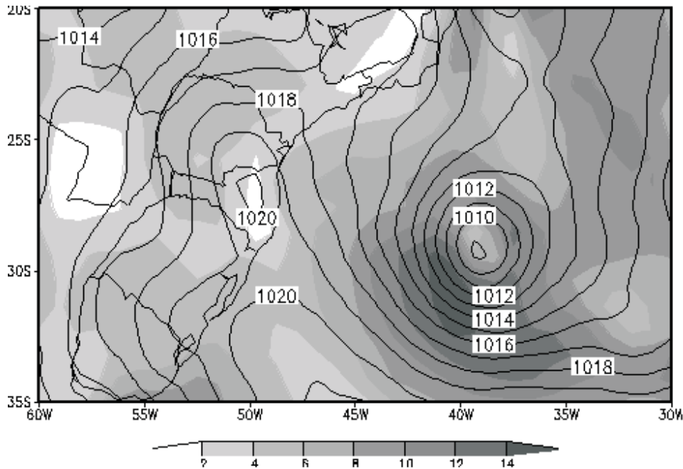
Figura 4.26 – Pressão ao nível médio do mar (hPa) (contornos) e velocidade do vento ( \text{m s}^{-1} ) (cores) sobre a região de atuação do ciclone Catarina para a condição inicial do NCEP de 24 de março de 2004 às 1200 UTC. A pressão no centro do ciclone é de cerca de 1008 hPa e os ventos mais intensos nas bordas dos sistema é de cerca de 14 \text{ m s}^{-1} .
