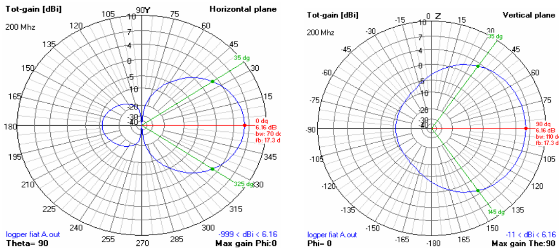
Figura 4.4-Diagrama de radiação para LPDA Básica em 200MHz.
